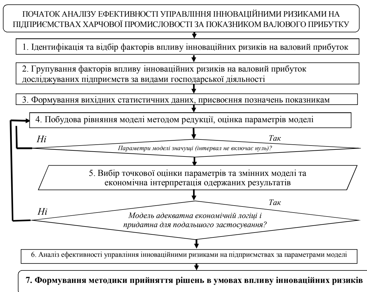
Рис. 3. Процедура аналізу ефективності управління інноваційними ризиками на підприємствах харчової промисловості із використанням багатofакторного моделювання валового прибутку.
