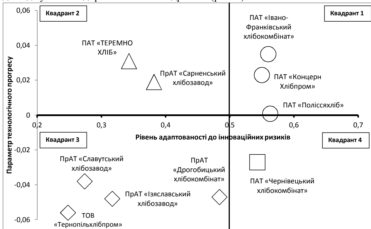
Рис. 5. Матриця «адаптованість до інноваційних ризиків – відповідність технологічному прогресу» хлібопекарських підприємств за 2001–2012 рр.
