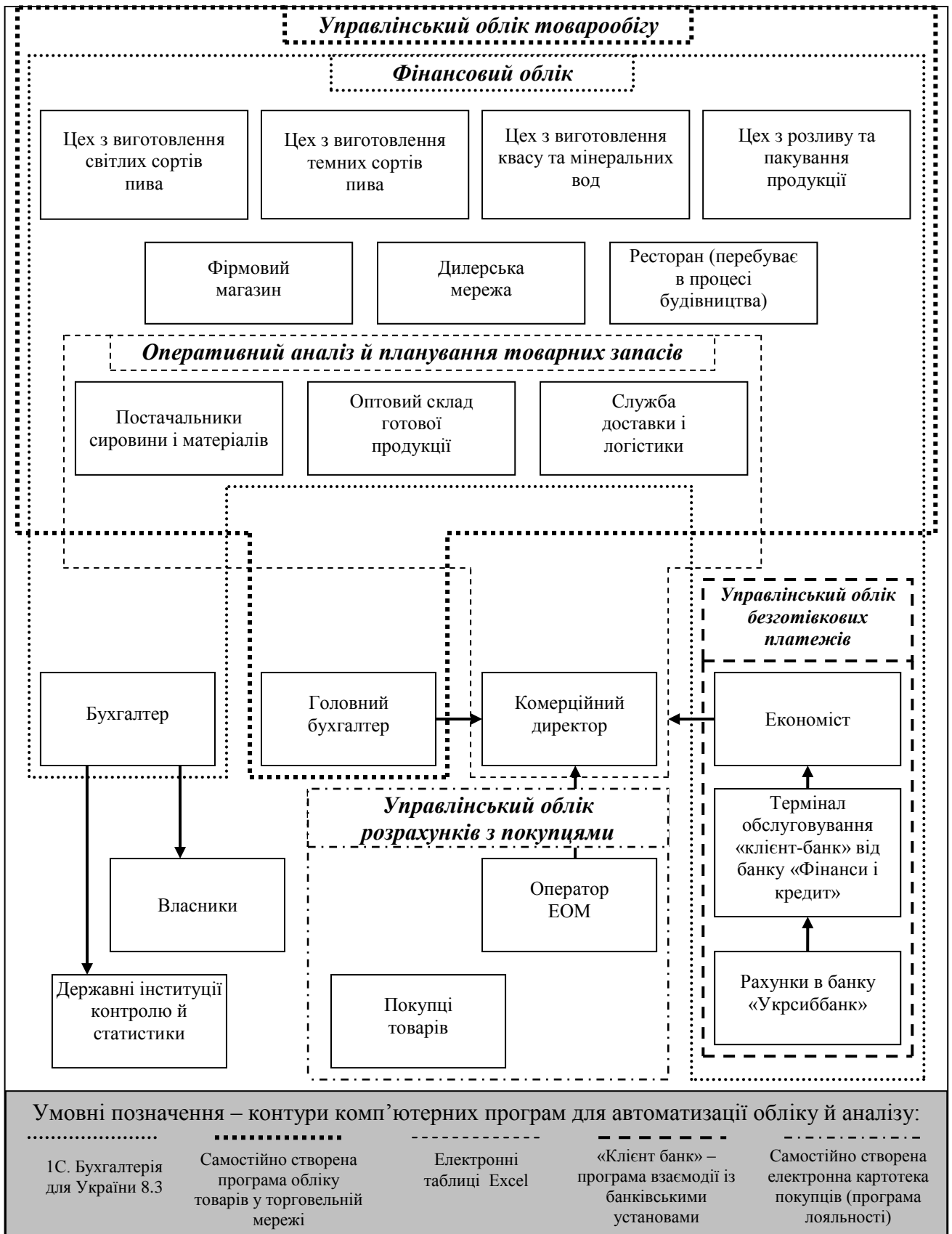
Рис. 5.1. Системи інформаційного супроводу діяльності ТОВ «Пивоварня «Опілля»
