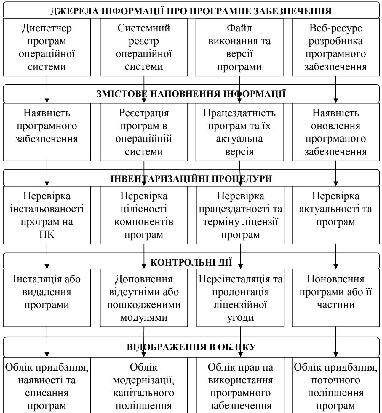
Рис. 3.3. Модель автоінвентаризації програмного забезпечення в умовах комп'ютерно-комунікаційної форми обліку
