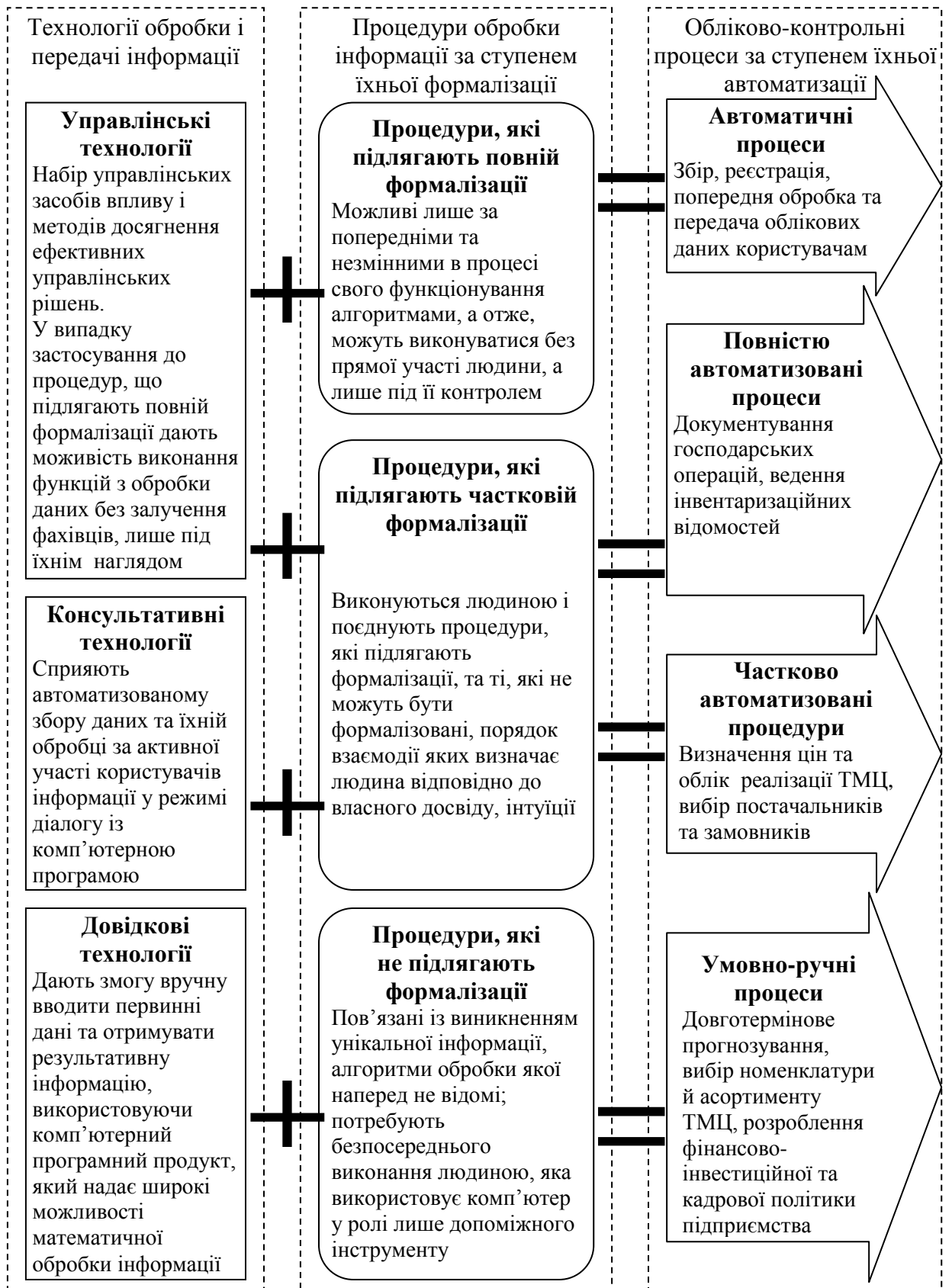
Рис. 1.12. Класифікація технологій обробки інформації та інформаційних процедур
