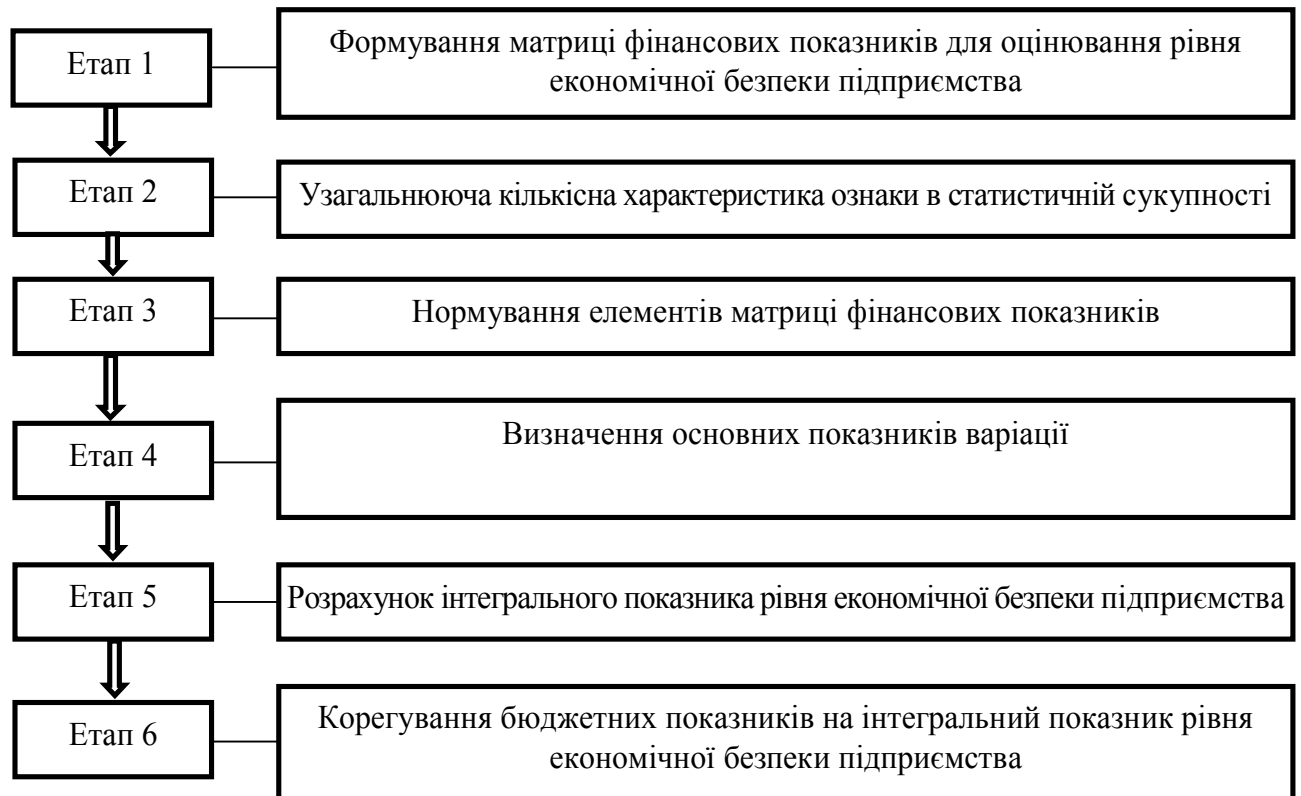
Рисунок 2.1 – Алгоритм інтегрального оцінювання рівня економічної безпеки підприємства
