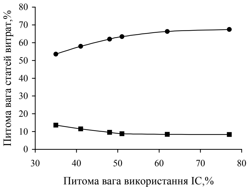
Рис. 2.3. Графік зміни питомих ваг вартості основних матеріалів і комплектуючих виробів – \Pi_M (графік 1) та заробітної плати – \Pi_3 (графік 2) у собівартості РЕА зі зміною процента використання ІС – \Pi_B .
