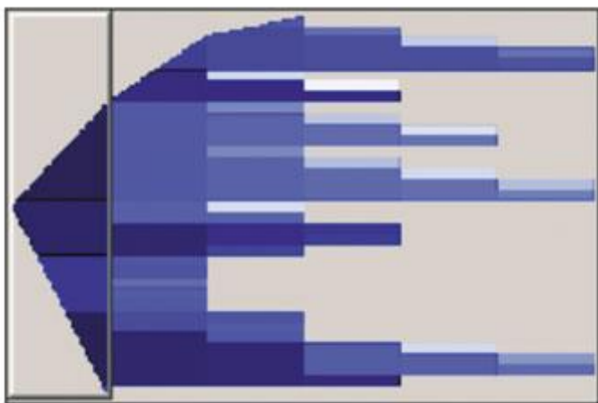
Рисунок 13. Дерево рішень.
