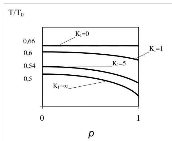
Рис.2. Графік розподілу температури в зоні контакту при різних значеннях коефіцієнта теплообміну K_1 = H_1 R .
