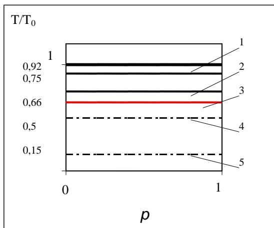
Рис.1. Графік розподілу температури в зоні контакту при різних значеннях контактної провідності h_0^1 : 1- h_0^{(1)}=0,1 ; 2- h_0^{(1)}=1 ; 3- h_0^{(1)}=\infty ; 4- h_0^{(1)}=1 ; 5- h_0^{(1)}=0,1 .
