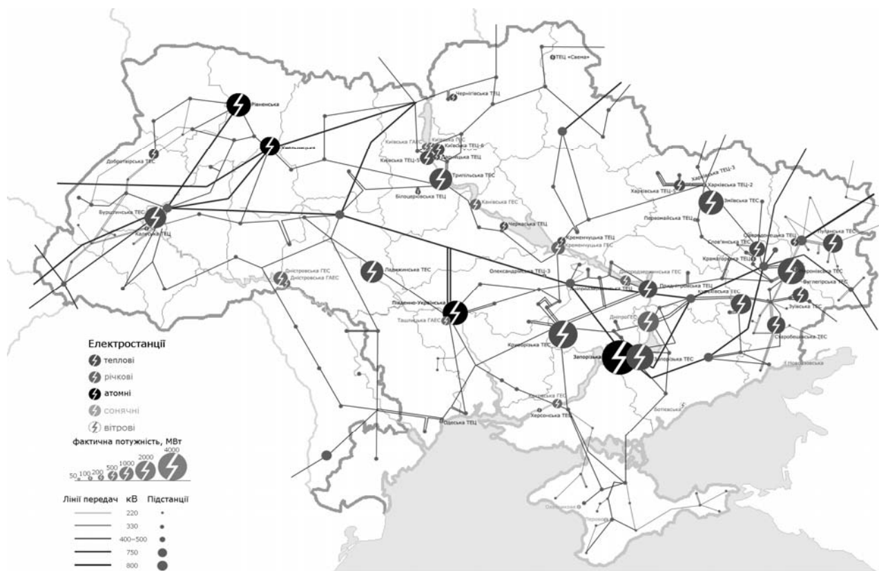
Рис. 10.5. Картошхема електростанцій України потужністю більше 50 МВт з лініями електропередачі та підстанціями
