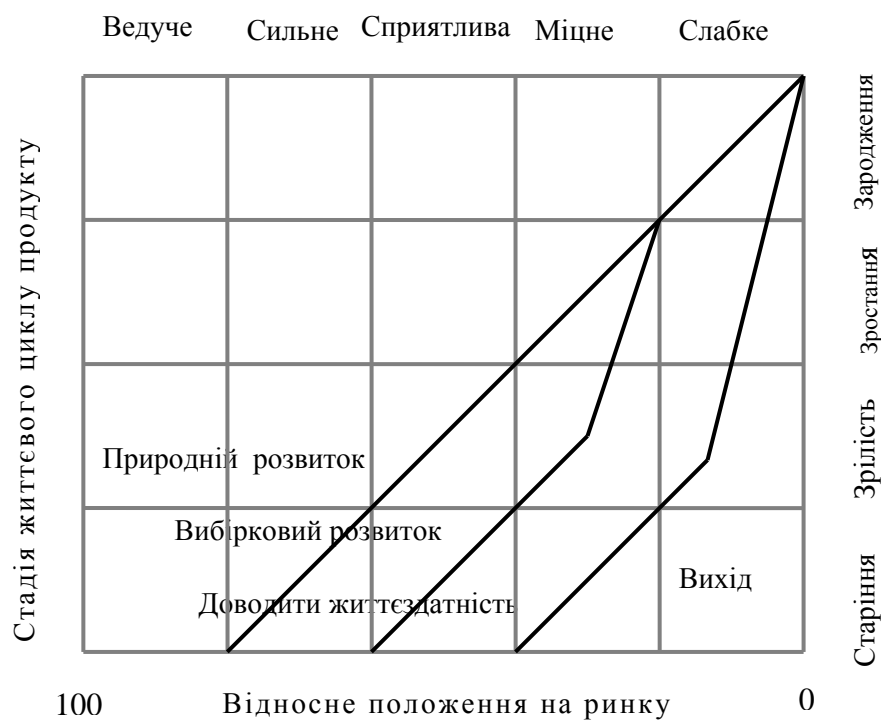
Рис.4 Матриця ADL/LC
