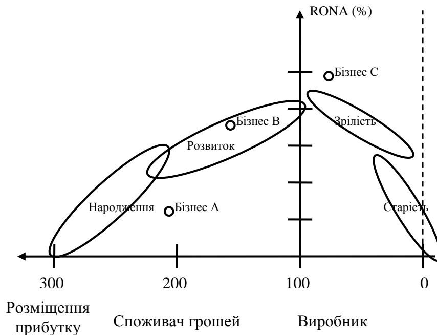
Рис.5 RONA - граф
