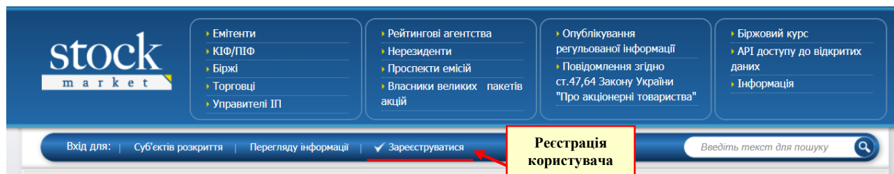
Рис. 1. Реєстрація користувача.
