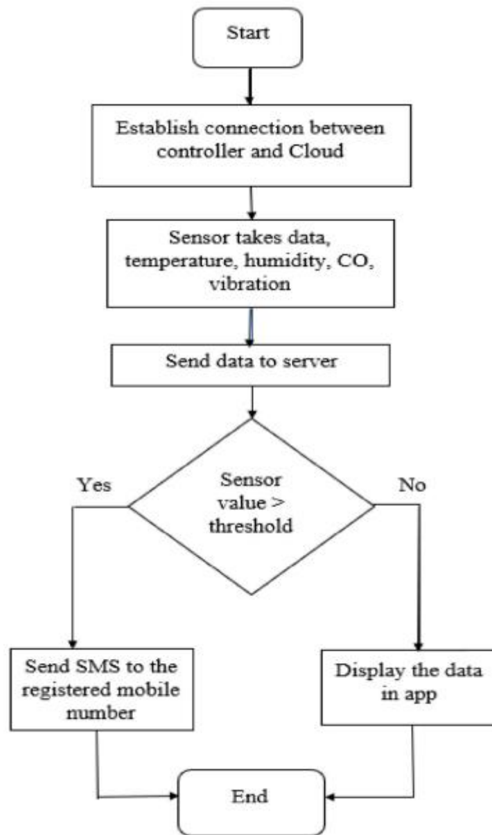
Рисунок 2.6 – Діаграма пропонованої системи
