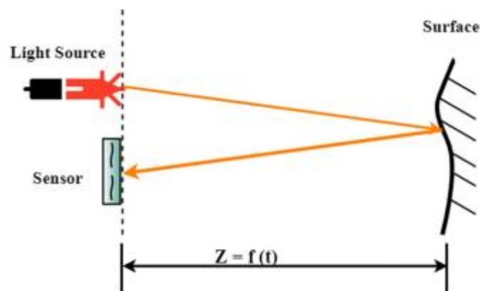
Рисунок 2.4 - Зображення через датчики TOF
