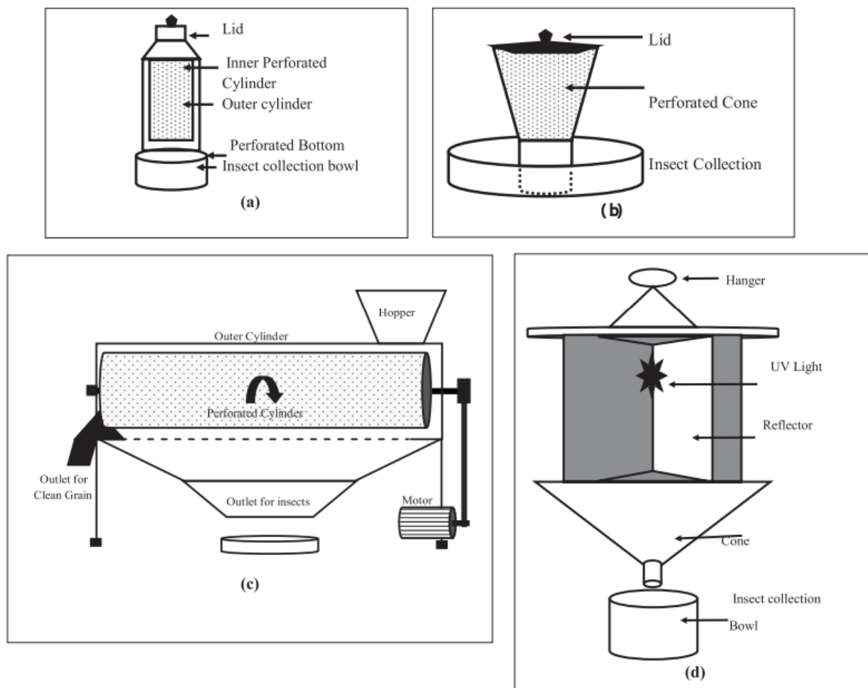
Рисунок 2.1 - (а) Пристрій-індикатор, (б) Бункер для автоматичного видалення комах, (с) Пристрій для видалення яєць комах, (д) Пастка ультрафіолетового світла.
