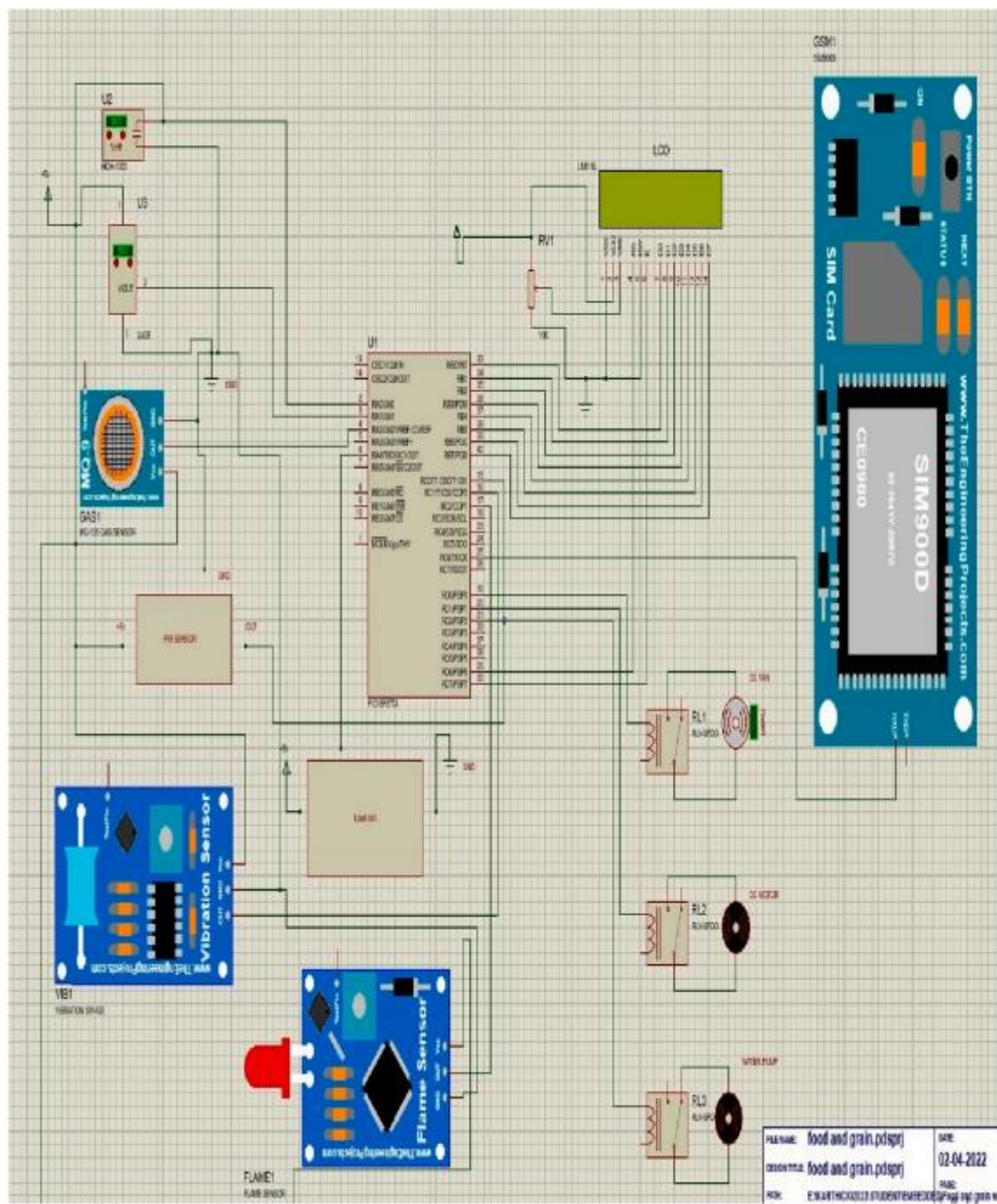
Рисунок 3.1 – змодельований апаратний склад модуля
