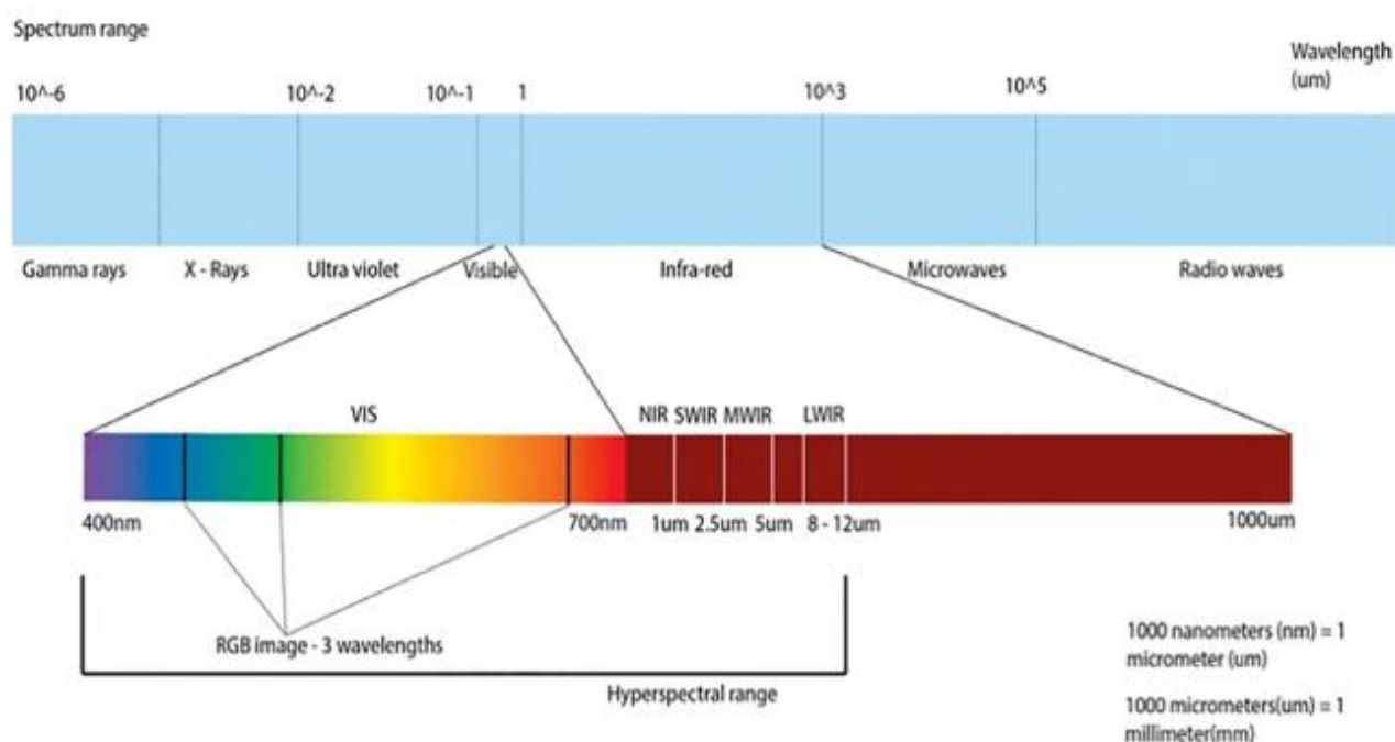
Рисунок 2.3 - Гіперспектральний діапазон в електромагнітному спектрі
