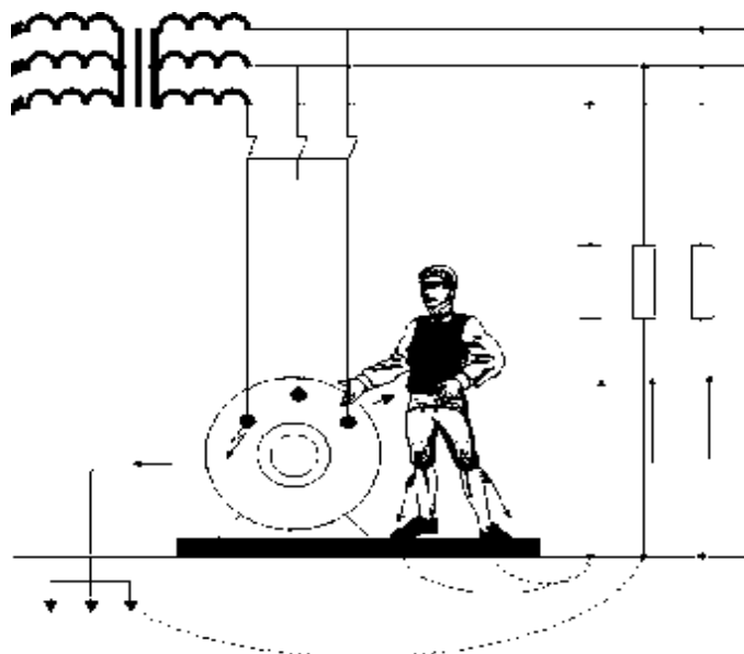
Рис. 3.7 – Схема захисного заземлення з ізолюованою нейтраллю
